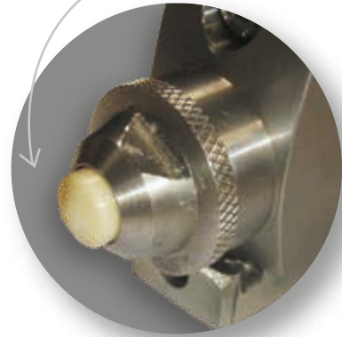
Gicleur équipé avec une tête en céramique
